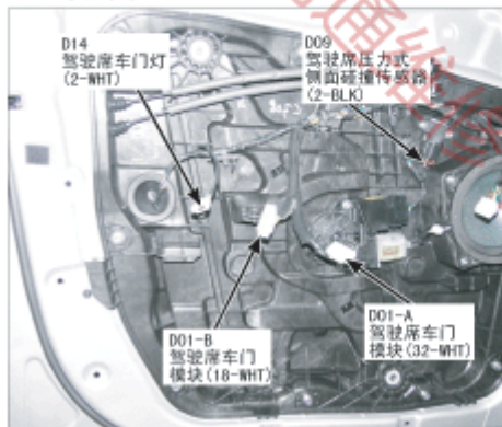
133. 驾驶席车门
